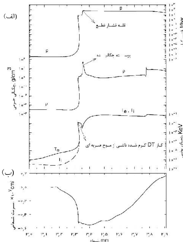
شکل ۹. نهشت انرژی راه‌انداز در لایه بیرونی و کنده شدن آن توسط نمایه شعاعی مقادیر هیدرودینامیکی در t=۰/۶ ns، (الف) دما، چگالی جرمی و فشار، (ب) سرعت سیال.
