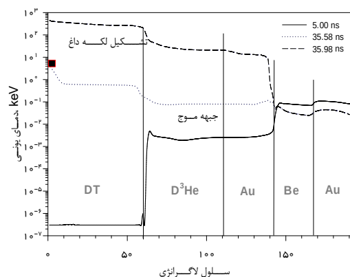
شکل ۶. دمای یونی لایه‌های هدف با پیکربندی سوخت \text{DT}+\text{D}^3\text{He} در سه مرحله مختلف تحول، (الف) در لحظه t=5/00 \text{ ns} پیش از بسته شدن حفره مرکزی، (ب) در لحظه t=35/58 \text{ ns} زمان تشکیل لکه داغ مرکزی و (پ) در لحظه t=35/98 \text{ ns} پایان فاز انفجار بیرونی.
