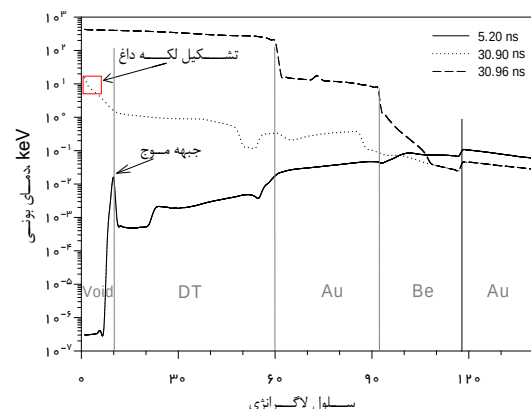
شکل ۴. دمای یونی لایه‌های هدف با سوخت DT خالص در سه مرحله مختلف تحول، (الف) در لحظه t=5/20 ns پیش از بسته شدن حفره مرکزی، (ب) در لحظه t=30/90 ns زمان تشکیل لکه داغ مرکزی و (پ) در لحظه t=30/96 ns پایان فاز انفجار بیرونی.
