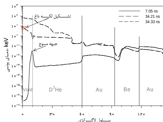
شکل ۴. دمای یونی لایه های هدف با سوخت D^+He خالص در سه مرحله مختلف تحول، (الف) در لحظه t=7/05 ns پیش از بسته شدن حفره مرکزی، (ب) در لحظه t=34/21 ns زمان تشکیل لکه داغ مرکزی و (پ) در لحظه t=34/33 ns پایان فاز انفجار بیرونی.
