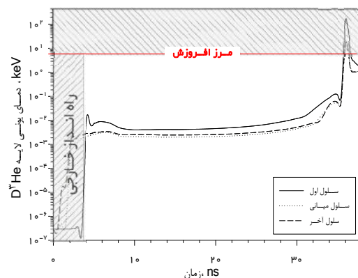
شکل ۷. (رنگی در نسخه الکترونیکی) تحول دمای یونی یاخته ابتدایی، میانی و انتهایی لایه سوخت D^3He در پیکربندی DT+D^3He (نوار قائم در محدوده زمانی ۰ تا ۳/۶ نانوثانیه، محدوده تابش باریکه خارجی و نوار افقی در بالا نشانگر محدوده دمایی افروزش است).
