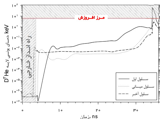
شکل ۳. (رنگی در نسخه الکترونیکی) تحول دمای یونی یاخته ابتدایی، میانی و انتهایی لایه سوخت D^+He خالص (نوار قائم در محدوده زمانی ۰ تا ۳/۶ نانو ثانیه، محدود تابش باریکه خارجی و نوار افقی در بالا نشانگر محدوده دمایی افروزش است).
