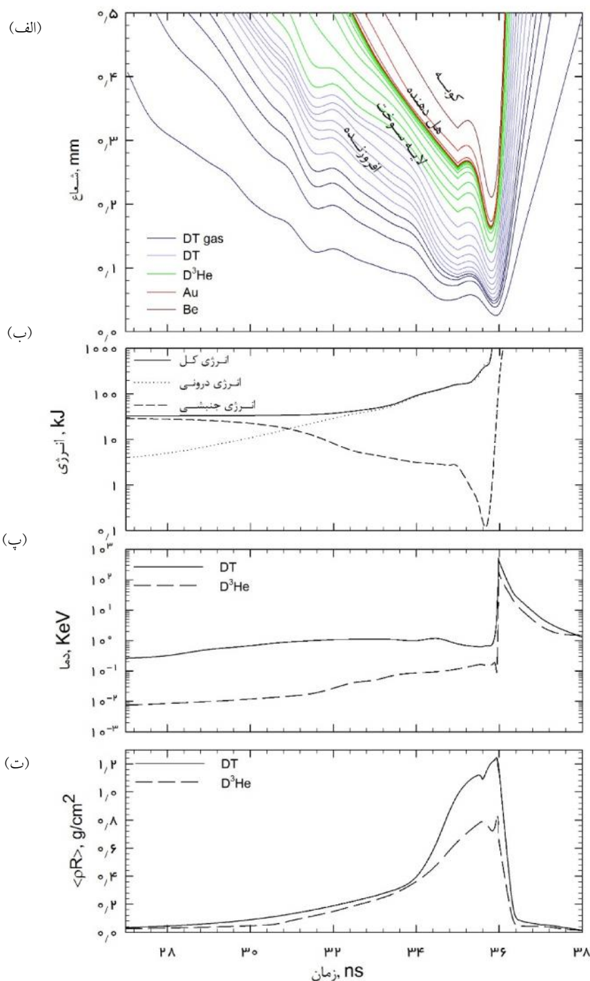
شکل ۱۱. (رنگی در نسخه الکترونیکی) کمیت‌های فیزیکی پیکربندی سوخت DT+D 3 He در زمان تشکیل لکه داغ مرکزی، (الف) شعاع، (ب) انرژی، (پ) دما و (ت) پارامتر محصورسازی \langle \rho R \rangle_{fuel} .
