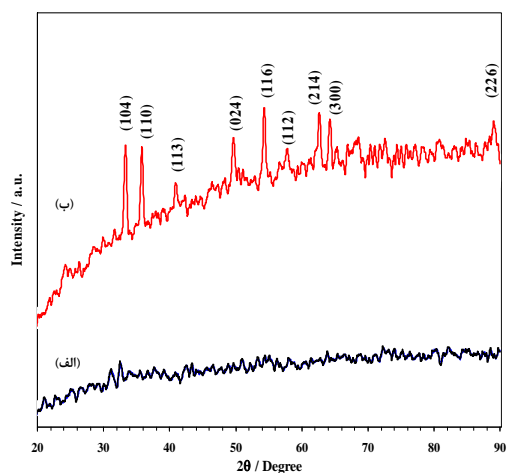
شکل ۳. (رنگی در نسخه الکترونیکی) نتایج آنالیز پراش پرتو ایکس برای نمونه‌های (الف) بلافاصله بعد ساخت و (ب) بعد از پخت.
