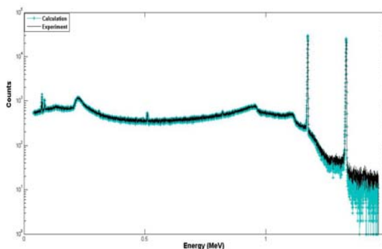
شکل ۳. (رنگی در نسخه الکترونیکی) مقایسه طیف کبالت -۶۰ حاصل از شبیه سازی با طیف تجربی معادل آن به ازای لایه مرده ای به ضخامت ۰,۵۷ mm.
