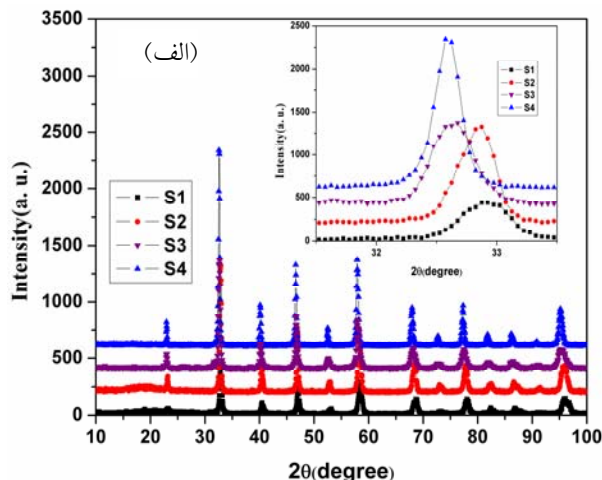
شکل ۱. (الف) طرح پراش پرتوی ایکس نمونه‌ها، شکل داخلی: جابه‌جایی قله‌ها با افزایش باریم (ب) طرح پراش پرتوی ایکس نمونه S4 همراه با تحلیل ریتولد آن.
