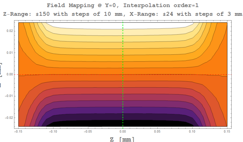
شکل ۱۰. نگاشت دوبعدی میدان مغناطیسی.
