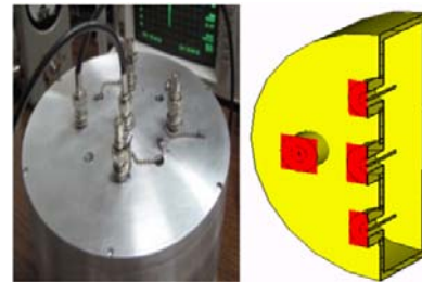
شکل ۱. ترکیب کننده توان ۴/۱ با محفظه استوانه‌ای.
