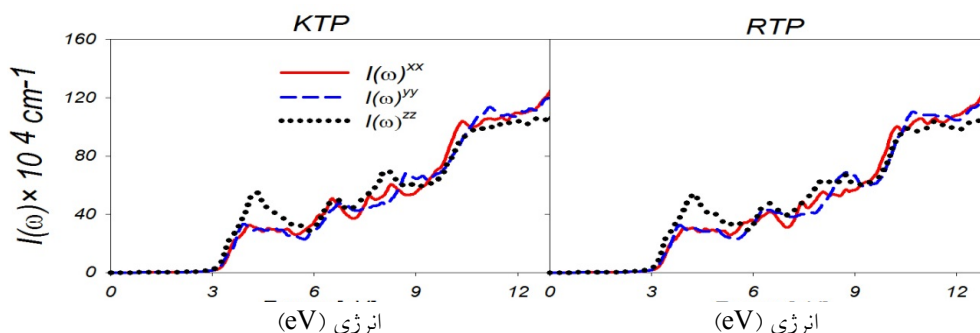
شکل ۹. (رنگی در نسخه الکترونیکی) نمودار طیف جذب KTP و RTP.
