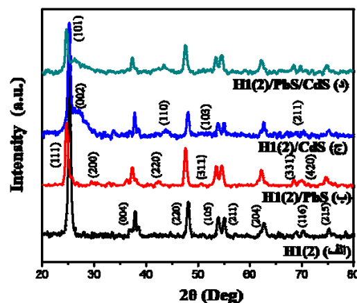
شکل ۴. (رنگی در نسخه الکترونیکی) طیف پراش پرتوی ایکس تهیه شده از فوتوآندهای (الف) H1(2) ، (ب) H1(2)/PbS ، (ج) H1(2)/PbS/CdS و (د) H1(2)/CdS .
