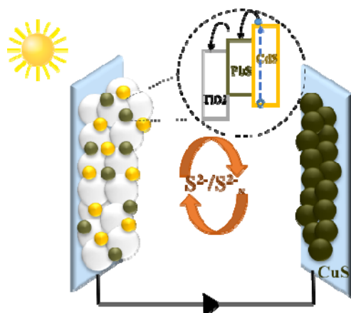
شکل ۱. (رنگی در نسخه الکترونیکی) نمایی از شکاف انرژی و انتقال‌های الکترونی نقاط کوانتومی PbS و CdS در یک سلول خورشیدی.
