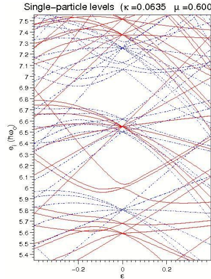
شکل ۱. (رنگی در نسخه الکترونیکی) ترازهای انرژی تک-ذره پروتونی در پتانسیل نیلسون با پارامترهای تک-ذره \kappa = 0.0635 و \mu' = 0.6 بر حسب پارامتر تغییر شکل چهار قطبی \mathcal{E} . خطوط پرنگ و خط چین به ترتیب نشان دهنده اوربیتال‌های با پاریته زوج و فرد هستند.
