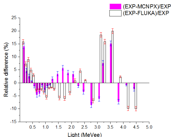
شکل ۱۰. (رنگی در نسخه الکترونیکی) اختلاف نسبی داده‌های شبیه‌سازی کدهای FLUKA، MCNPX با داده‌های تجربی، برای آشکارساز سوسوزن A ۵۰۱ BC با هندسه استوانه‌ای و ابعاد ۲"×۲" که در معرض چشمه نوترونی ^{241}\text{Am-Be} قرار گرفته است.
