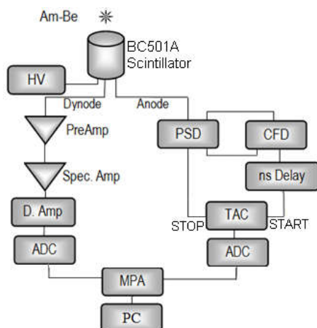
شکل ۳. چیدمان آزمایش جدا سازی نوترون-گاما به روش گذر از صفر.
