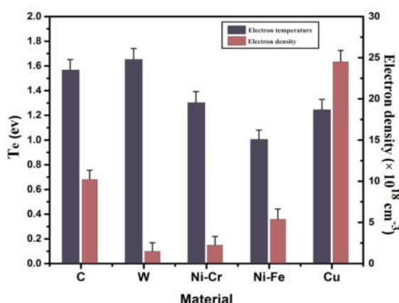
شکل ۷. دما و چگالی الکترونی به دست آمده برای آنتن‌های مختلف برای گوی پلاسمایی.
