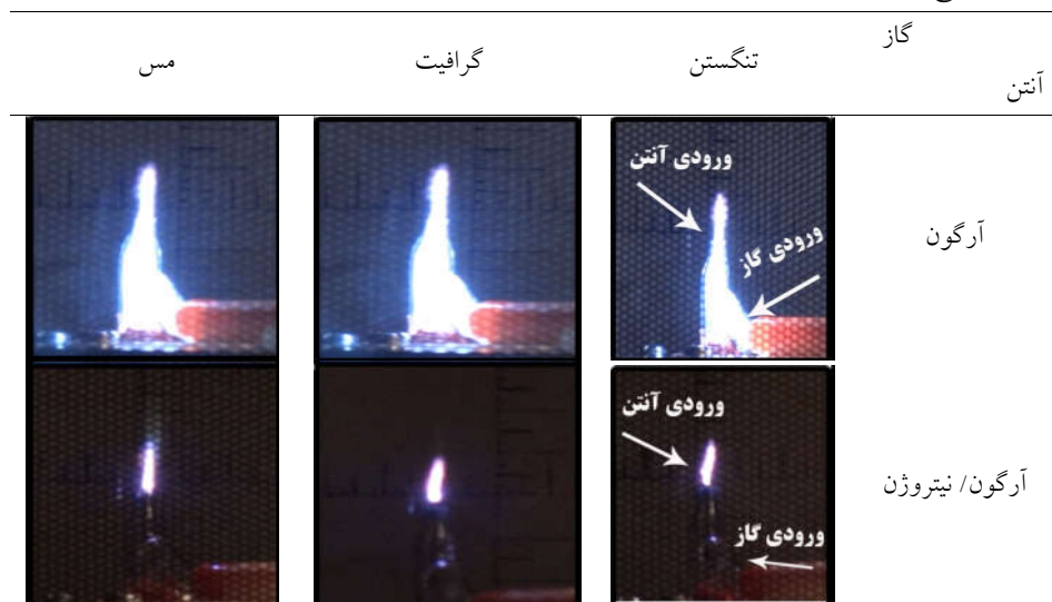
جدول ۲. جت پلاسمای موج میکرو تولید شده در مجاورت گاز آرگون و آرگون/ نیتروژن.
