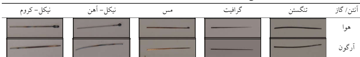
جدول ۳. تصویر آنتن‌های گوی پلاسمای موج میکرو در مجاورت هوا و گاز آرگون بعد از تولید پلاسما.
