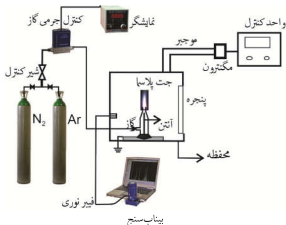
شکل ۳. چیدمان آزمایش جت پلاسما موج میکرو در فشار اتمسفری.
