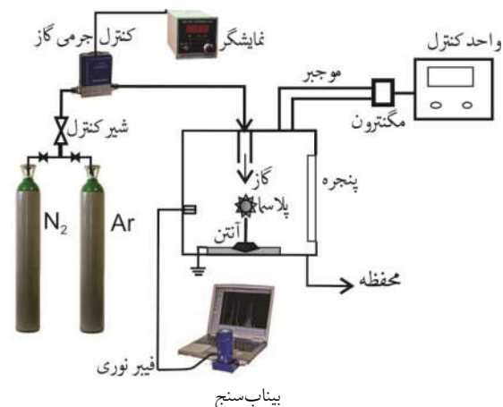
شکل ۲. چیدمان آزمایش گوی پلاسما موج میکرو در فشار اتمسفری.
