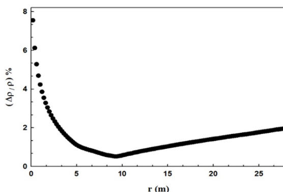
شکل ۶. نمودار خطای نسبی چگالی تعداد ذرات محاسبه شده با تابع توزیع NKG برای \beta عدد ۵۰ بر حسب فاصله از هسته برای یک بهمن هوایی عمودی پروتون با انرژی ۳۰۰ TeV.
