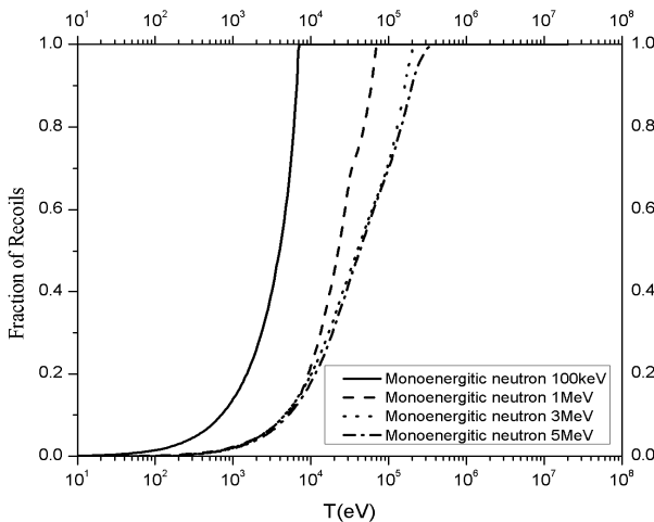
شکل ۵. طیف اتم‌های پس زده اولیه نوترون‌های تک انرژی با انرژی‌های ۱۰۰ keV، ۱ MeV، ۳ MeV، ۵ MeV، بر روی هدف ۵۶ Fe.
