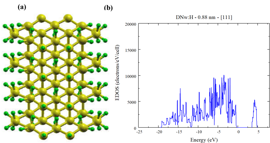
شکل ۵. سطح جانبی (a) و چگالی حالت‌های الکترونی (b) نانوسیم الماس اشباع شده با قطر 0.88 \text{ nm} رشد یافته در جهت (۱۱۱).
