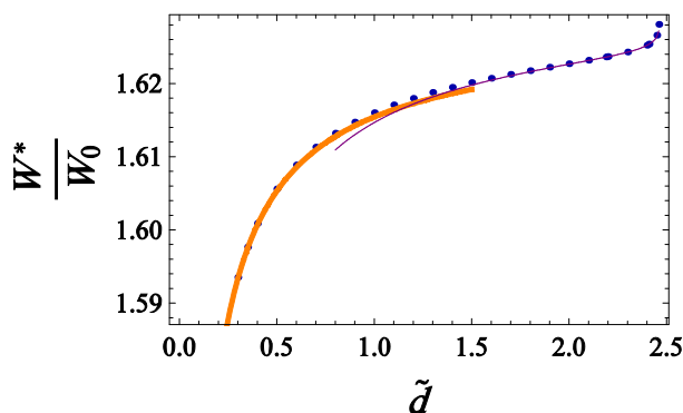
شکل ۱. (رنگی در نسخه الکترونیکی) مقادیر عددی نسبت شدت مؤثر برهم کنش بر شدت میانگین (\frac{W^*}{W_0} = 1 - \Lambda^*) بر حسب فاصله بی بعد \tilde{d} = d/\lambda به ازای \lambda/a = 100 و \chi = 0.002 در رابطه (۱۴). منحنی‌های ضخیم و نازک به ترتیب مربوط به جواب‌های تحلیلی صادق در فواصل کوچک رابطه (۱۶) و فواصل بزرگ رابطه (۱۹) هستند.
