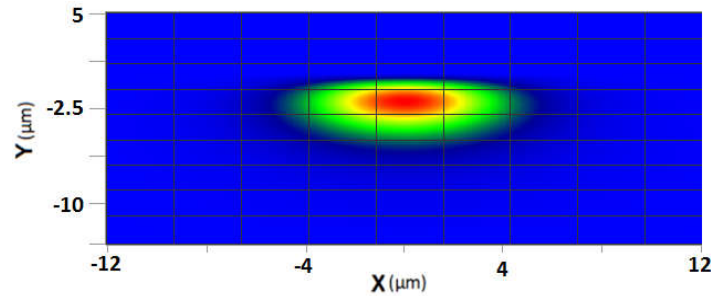
شکل ۲. (رنگی در نسخه الکترونیکی) مد نور موجبر با عرض پوشش 6\mu\text{m} با تبادل پروتون یک ساعت در دمای 170^\circ\text{C} درجه و بازپخت ۵ ساعت در دمای 375^\circ\text{C} درجه در طول موج 1550\text{nm} .
