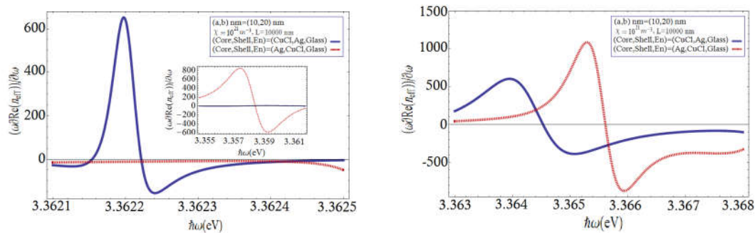
شکل ۴. (رنگی در نسخه الکترونیکی) بررسی جنس هسته و پوسته نانوذره بر میزان کاهش سرعت نور در نانوذرات استوانه‌ای هسته- پوسته تزریق شده در محیطی با ثابت دی‌الکتریک \epsilon_r = ۲/۲۵ با فرض \chi = 10^{21} m^{-3} و \mathcal{N} = ۱۰^{۲۱} m^{-3} و b = ۲۰ nm و a = ۱۰ nm
