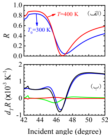
شکل ۳. (رنگی در نسخه الکترونیکی) (الف) ضریب بازتاب حسگر شکل ۱ در دو دمای ۳۰۰ و ۴۰۰ کلوین، (ب) تغییرات گرمایی ضریب بازتاب dTR (منحنی سیاه) و سهم خواص گرما-نوری فلز طلا (منحنی آبی)، منشور (منحنی سبز) و محیط حسگری (منحنی قرمز) در dTR .
