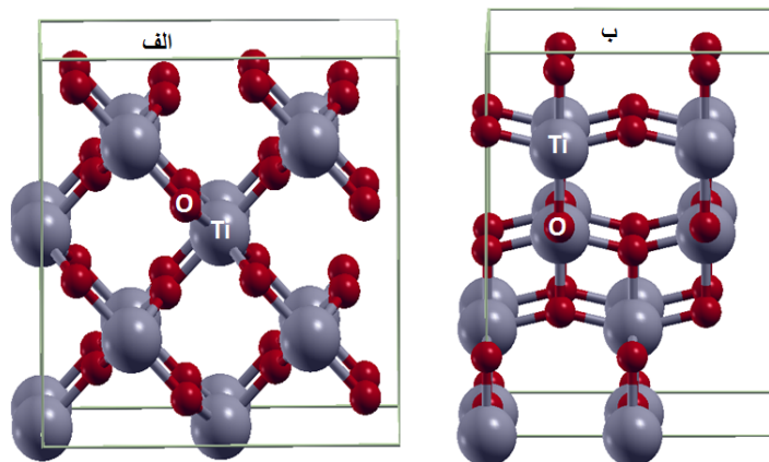
شکل ۱. (رنگی در نسخه الکترونیکی) ساختار بلوری مدل محاسبه‌ای ابرباخته ۴۸ اتمی، (الف) روتیل و (ب) آناز. (رنگی در نسخه الکترونیکی)
