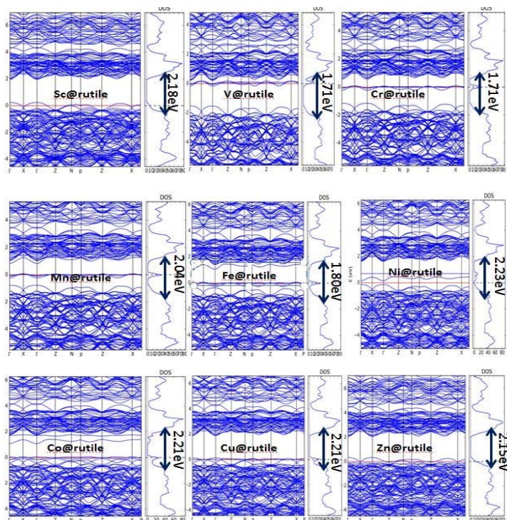
شکل ۴. (رنگی در نسخه الکترونیکی) چگالی حالت‌های الکترونی کل و ساختار نواری روتیل آلاینده با فلزهای واسطه. خط قرمز تراز فرمی را نشان می‌دهد.
