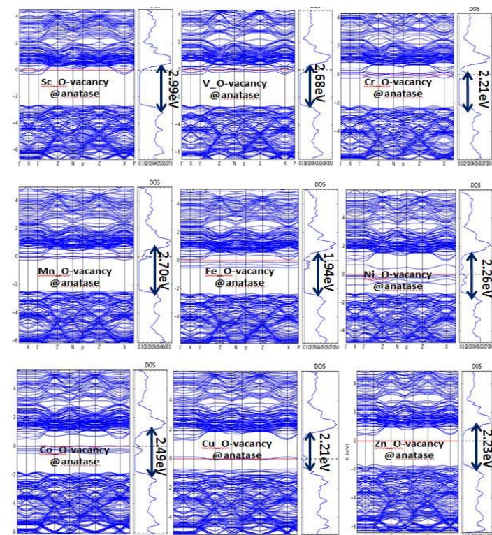
شکل ۷. (رنگی در نسخه الکترونیکی) چگالی حالت‌های الکترونی کل و ساختار نواری آناتاز آلاینده با فلز واسطه و همراه با نقص تهی‌جای اکسیژن. خط قرمز تراز فرمی را نشان می‌دهد.
