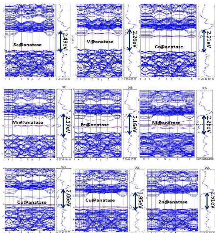
شکل ۵. (رنگی در نسخه الکترونیکی) چگالی حالت‌های الکترونی کل و ساختار نواری آناتاز آلاینده با فلزهای واسطه. خط قرمز تراز فرمی را نشان می‌دهد.
