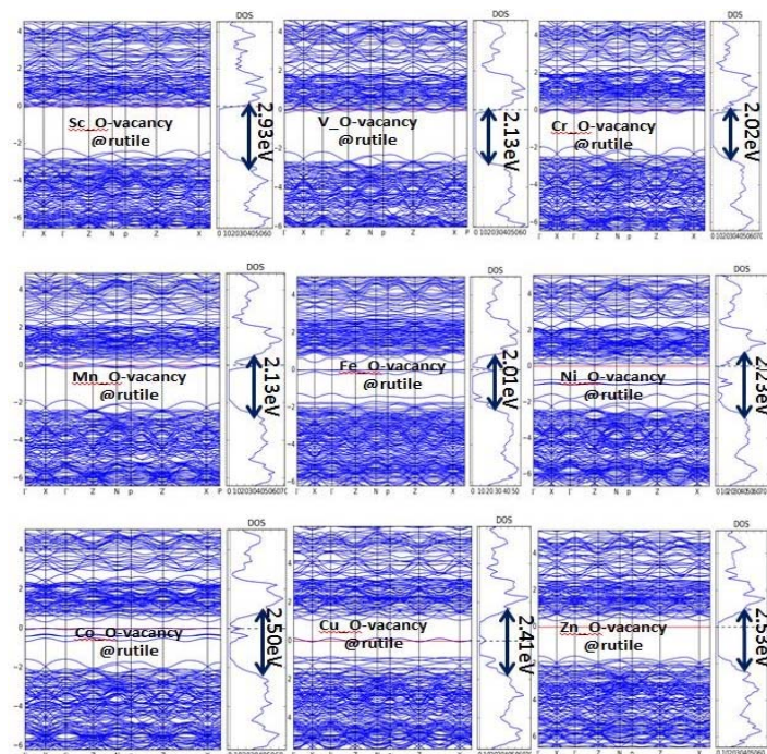
شکل ۶. (رنگی در نسخه الکترونیکی) چگالی حالت‌های الکترونی کل و ساختار نواری روتیل آلاینده با فلز واسطه و همراه با نقص تهی‌جای اکسیژن. خط قرمز تراز فرمی را نشان می‌دهد.
