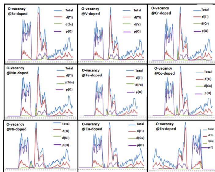
شکل ۹. (رنگی در نسخه الکترونیکی) چگالی حالت‌های الکترونی جزئی آنتاز آلائیده با فلز واسطه و همراه با نقص تهی جای اکسیژن.
