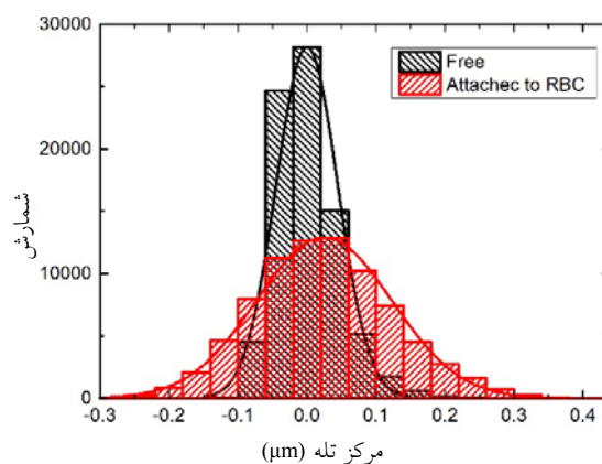
شکل ۸. (رنگی در نسخه الکترونیکی) نمودار فراوانی مکان ذره نسبت به مرکز تله در حالت آزاد (سیاه) و حالت متصل به گلبول (قرمز).
