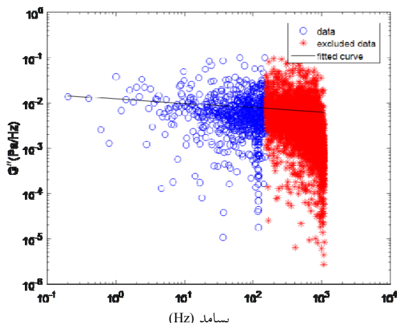
شکل ۱۰. (رنگی در نسخه الکتریکی) نمودار مدول اتلافی تقسیم بر حسب بسامد آب برای ذره‌ای به قطر دو میکرومتر.
