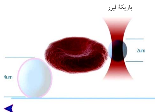
شکل ۱. (رنگی در نسخه الکترونیکی) میکروکره چهار میکرومتری بر روی لامل به عنوان پایه قرار گرفته و میکروکره دو میکرومتری با استفاده از انبرک نوری به دام افتاده است و گلبول از دو انتها به دو میکروکره متصل شده است.
