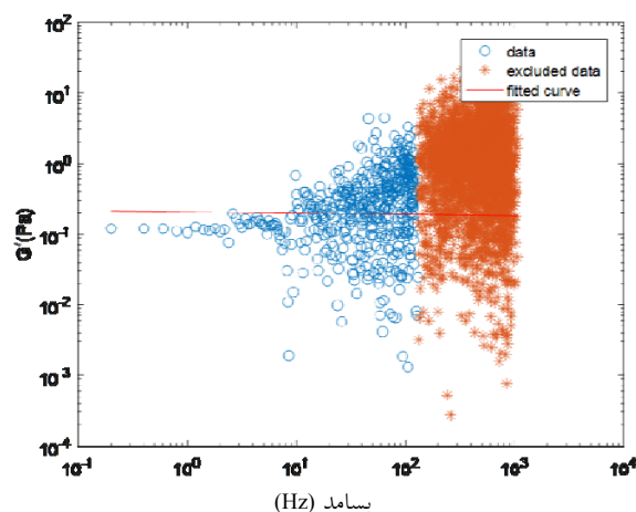
شکل ۹. (رنگی در نسخه الکتریکی) نمودار مدول کشسانی آب بر حسب بسامد که به خوبی عدم وابستگی آن را به بسامد نشان می‌دهد. قسمت‌های نارنجی داده‌های جدا شده هستند و خط قرمز شیب برازش شده به نمودار در بسامدهای پایین است.
