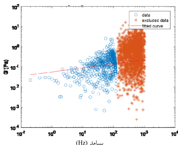
شکل ۱۱. (رنگی در نسخه الکترونیک) نمودار مدول کشسانی میکروکره متصل به گلبول.
