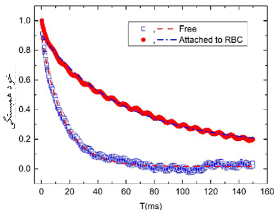
شکل ۷. (رنگی در نسخه الکترونیکی) تابع خود همبستگی ذره در تله نوری در حالت آزاد (آبی) و متصل به گلبول (قرمز).
