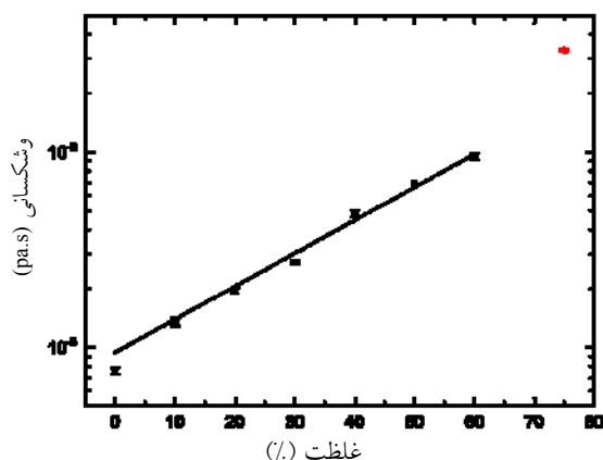
شکل ۴. (رنگی در نسخه الکترونیکی) نمودار نشان دهنده تغییرات وشکسانی با غلظت مخلوط آب و گلیسرین است. که نقاط به ترتیب ۰٪، ۱۰٪، ۲۰٪، ۳۰٪، ۴۰٪، ۵۰٪، ۶۰٪ و ۷۵٪ است.
