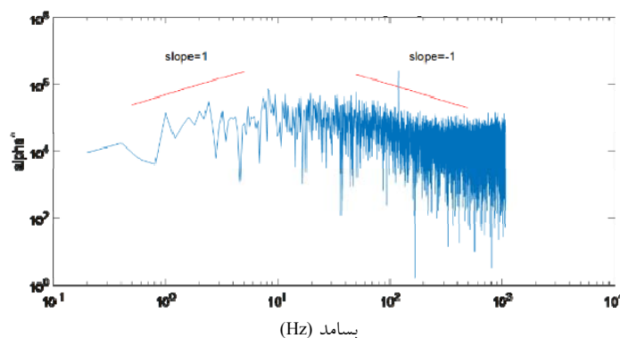
شکل ۹. (رنگی در نسخه الکترونیکی) نمودار تابع \alpha'' بر حسب بسامد.
