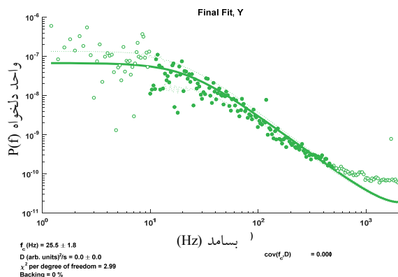
شکل ۲. (رنگی در نسخه الکترونیکی) برازش منحنی لورنتزی به داده‌های میکروکره دو میکرومتری برای محاسبه سختی تله و روش تحلیلی طیف توانی.
