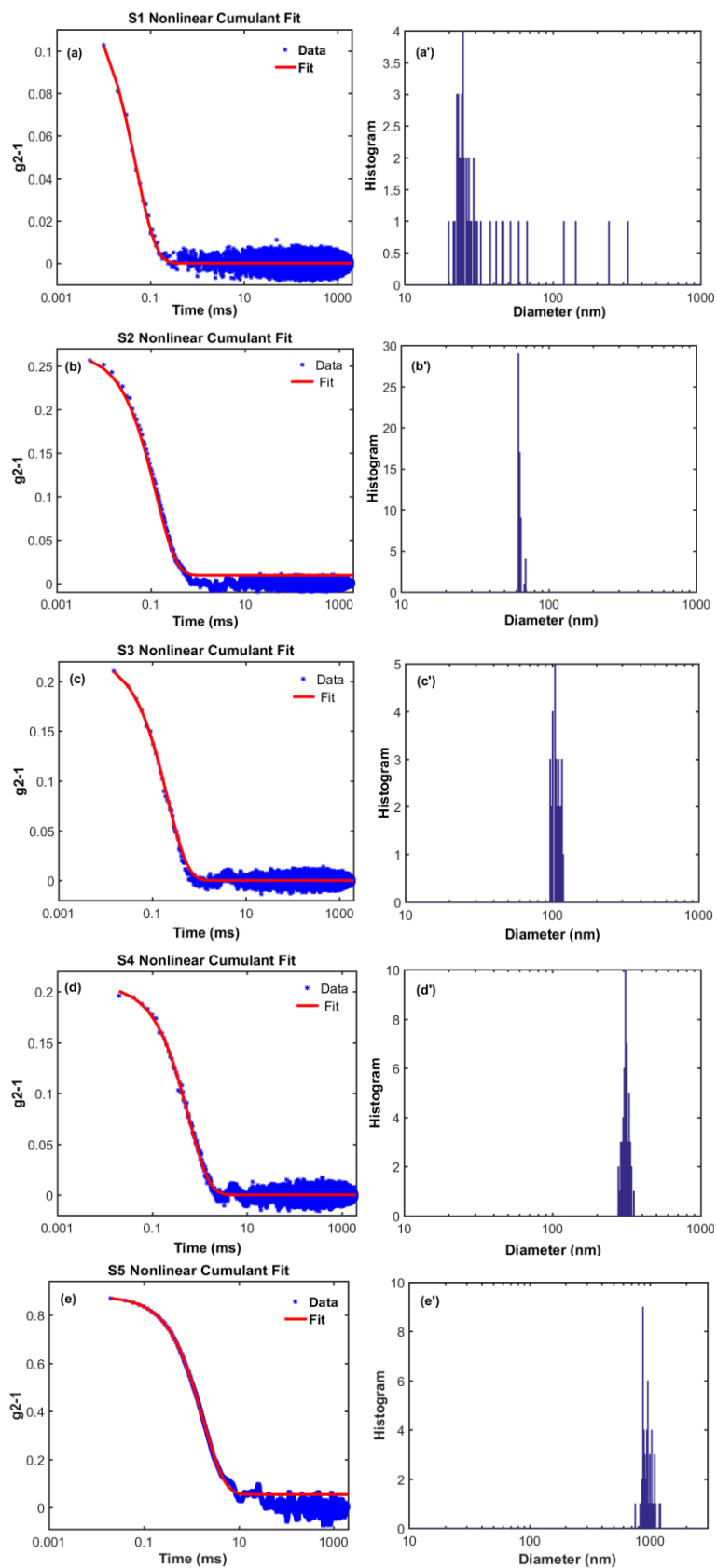
شکل ۲. (رنگی در نسخه الکترونیکی) (e)-(a) نمودار تابع خودهمبستگی شدت (نقاط) و برازش داده‌های تجربی به رابطه (۱۱) (خط توپر) بر حسب زمان به ترتیب برای نمونه‌های S۵-S۱. (e')-(a') نمودار فراوانی اندازه ذرات به ترتیب متناظر با (e)-(a).
