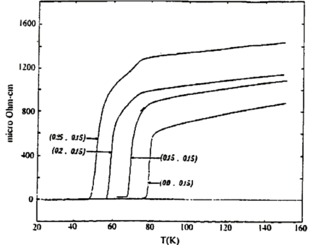
شکل ۳. منحنی مقاومت ویژه برحسب دما نمونه‌های GdPrCa-123 با غلظت ثابت یون Ca (۱۵٪) و با مقادیر متفاوت یون Pr 0/25 ، 0/1 ، 0/15 ، 0/2 .
