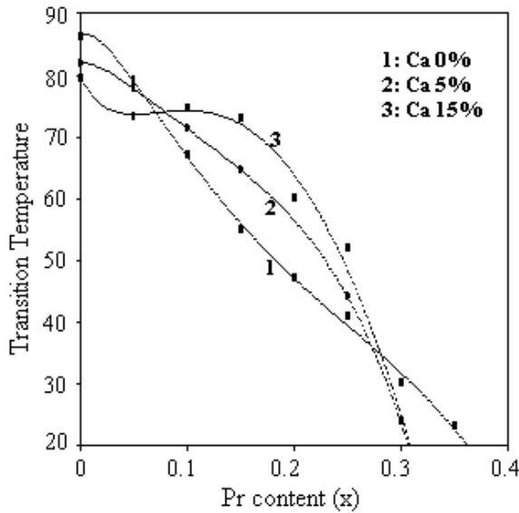
شکل ۵. منحنی دمای گذار برحسب غلظت یون Pr در نمونه‌های GdPrCa-123 . (الف) Ca 0\% ، (ب) Ca 10\% ، (ج) Ca 15\% خطوط راهنمای چشم‌انداز. نقاط شکل (الف) از مرجع [۲۱] اخذ شده‌اند.
