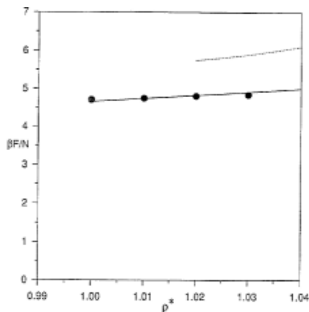
شکل ۳. انرژی آزاد هلمهولتز بر واحد ذره بلور fcc برحسب چگالی کپه‌ای کاهش یافته، خط ممتد مربوط به شبیه‌سازی مونت-کارلو، دایره‌های توپر مربوط به محاسبات انجام شده با در نظر گرفتن تابع همبسته مستقیم GMSA و نقطه‌چین مربوط به تابع همبسته مستقیم PY می‌باشند.
