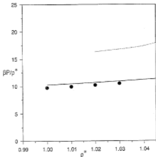
شکل ۴. معادله حالت بلور fcc، خط ممتد مربوط به شبیه‌سازی مونت-کارلو، دایره‌های توپر با در نظر گرفتن تابع همبسته مستقیم GMSA و نقطه‌چین مربوط به تابع همبسته مستقیم PY می‌باشد.
