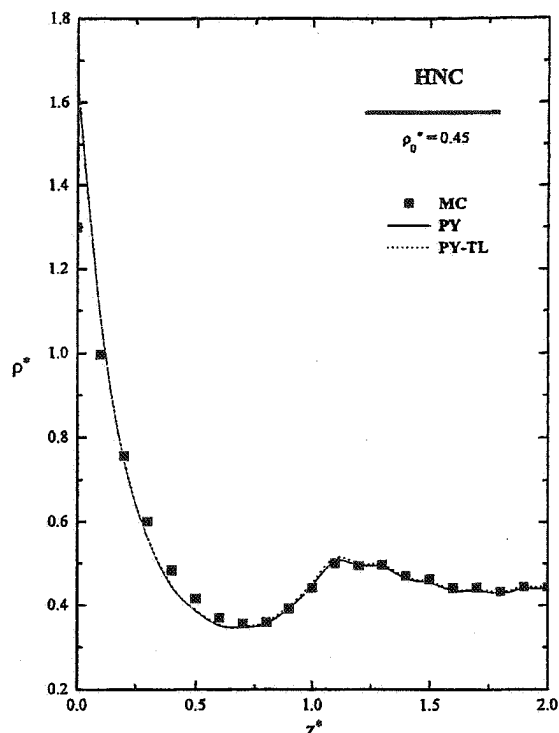
شکل ۳. چگالی مدل مایع کره سخت برحسب فاصله کاهش یافته از دیواره سخت ( z^* = z/\sigma ) که از حل معادله انتگرالی غیرخطی HNC در چگالی کاهش یافته \rho^* = 0.45 نتیجه شده است. نقاط مربعی مربوط به نتایج شبیه سازی کامپیوتری، منحنی ممتد مربوط به به کار بردن تابع همبستگی تقریب PY و منحنی خط چین با استفاده از تابع همبستگی مستقیم دنباله دار می‌باشد.
