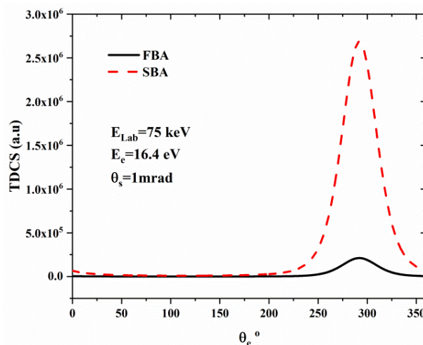
شکل ۲. (رنگی در نسخه الکترونیکی) مقایسه سطح مقطع سه‌گانه تقریب‌های مرتبه اول و دوم بورن برای یونش اتم هیدروژن در برخورد با پروتون با انرژی فرودی ۷۵ keV و الکترون آزاد شده با انرژی ۱۶/۴ eV در زاویه پراکندگی \theta_s = 1 \text{ mrad} .
