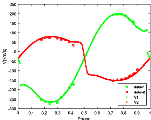
شکل ۱۱. (رنگی در نسخه الکترونیکی) منحنی‌های مشاهده‌ای و محاسباتی سرعت‌های شعاعی ستارگان اولیه و ثانویه بر حسب فاز دستگاه دوتایی BD+۴۲۲۷۸۲. داده‌های مشاهده‌ای از [۱۱] است.
