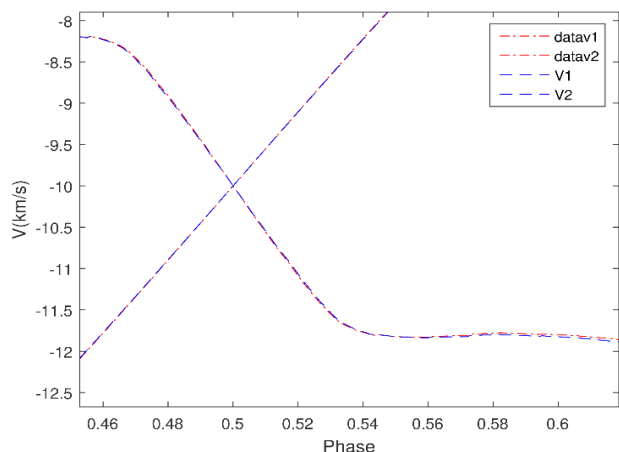
شکل ۶. (رنگی در نسخه الکترونیکی) منحنی‌های سرعت شعاعی دستگاه نمونه که درشت‌نمایی شده بر حسب فاز در اطراف فاز ۰.۵ رسم شده‌اند. datav_1 و datav_2 منحنی‌های سرعت شعاعی دستگاه نمونه برای ضرایب روشنایی سطحی دقیق محاسبه شده هستند، و V_1 و V_2 منحنی‌های سرعت شعاعی با ضرایب روشنایی سطحی به دست آمده از طیف سنجی هستند.
