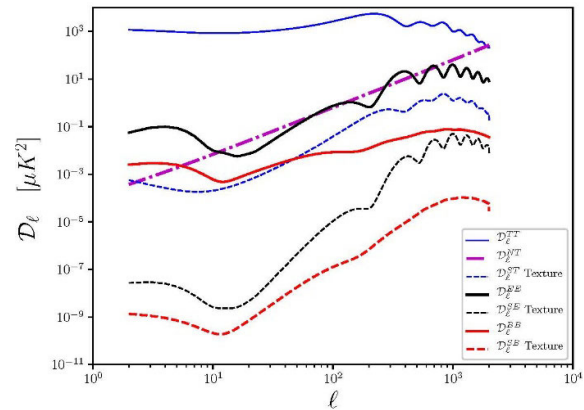
شکل ۳. (رنگی در نسخه الکترونیکی) طیف توان کیمتهای مختلف به همراه طیف توان چشمه ناشی از اثر همگرایی گرانشی مدل بافت کیهانی برای لکه سرد.
