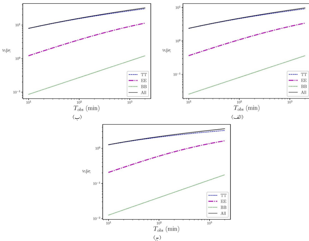
شکل ۴. (الف) نسبت سیگنال به نوفه بر حسب مدت زمان رصد ناشی از اثر همگرایی گرانشی مدل تهی‌جا برای لکه سرد با تباین چگالی \delta = -0.3 . (ب) همانند بخش بالا به جز برای تباین چگالی \delta = -0.7 . (ج) نسبت سیگنال به نوفه بر حسب مدت زمان رصد ناشی از اثر همگرایی گرانشی مدل بافت کیهانی برای لکه سرد.
