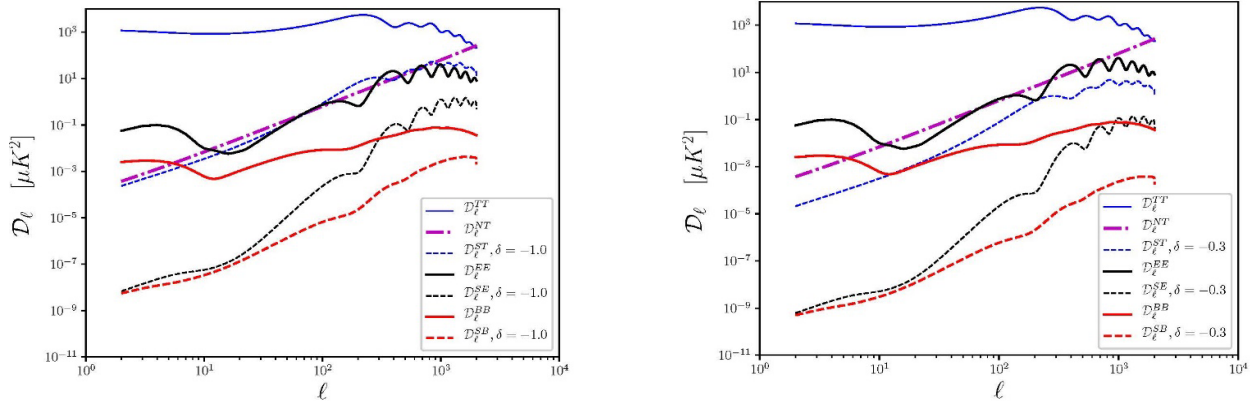
شکل ۲. (رنگی در نسخه الکترونیکی) طیف توان کیمتهای مختلف به همراه طیف توان چشمه ناشی از اثر همگرایی گرانشی مدل تهی جا برای لکه سرد با تباین چگالی \delta = -0.3 . چپ: همانند شکل سمت راست به جز برای تباین چگالی \delta = -1.0 .
