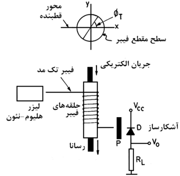
شکل ۱۳. حسگر فیبرنوری برای اندازه گیری جریان الکتریکی.
