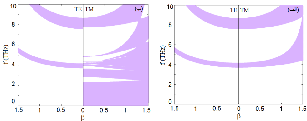
شکل ۳. (رنگی در نسخه الکترونیکی) باندهای عبور و ممنوعه بلور فوتونی برای قطبش های TE و TM برای حالت های (الف) \varphi = 0^\circ و (ب) \varphi = 3^\circ . نواحی روشن نشانگر باندهای ممنوعه و نواحی تیره نشانگر باندهای عبور هستند. در این نمودار T = 300\text{ K} و \mu_c = 0.25\text{ eV} در نظر گرفته شده است.
