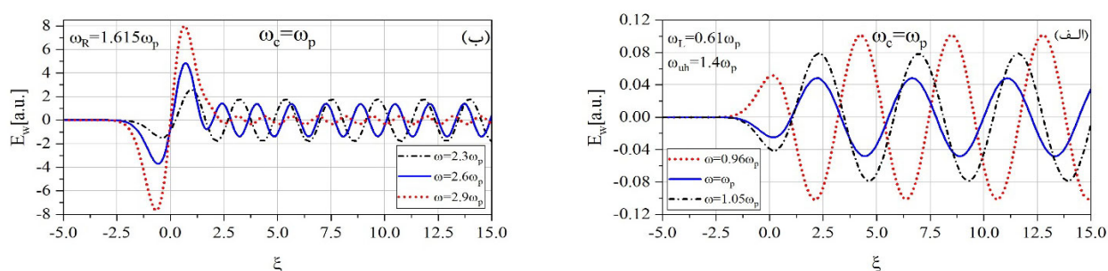
شکل ۱۱. (رنگی در نسخه الکترونیکی) دامنه میدان دنباله برای مُد X به ازای \omega_c = \omega_p . (الف) ناحیه انتشار اول و (ب) ناحیه انتشار دوم.
