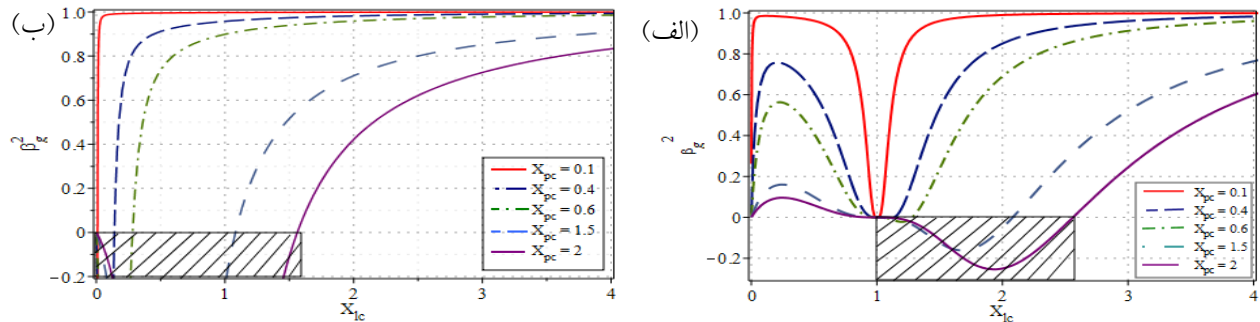
شکل ۲. (رنگی در نسخه الکترونیکی) تغییرات \beta_g^2 نسبت به X_{lc} با مقادیر ثابت X_{pc} (الف) \sigma = +1 و (ب) \sigma = -1 .
