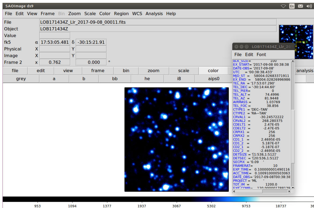
شکل ۱. (رنگی در نسخه الکترونیکی) نمونه‌ای از یک تصویر نجومی که به کمک نرم‌افزار ds9 باز شده است. فایل سر فصل که حاوی تمامی مشخصات تصویر است نیز در سمت راست آمده است. این تصویر به کمک تلسکوپ ۱/۵ متری دانمارک و به وسیله دوربین تصویر برداری شانس گرفته شده است.
