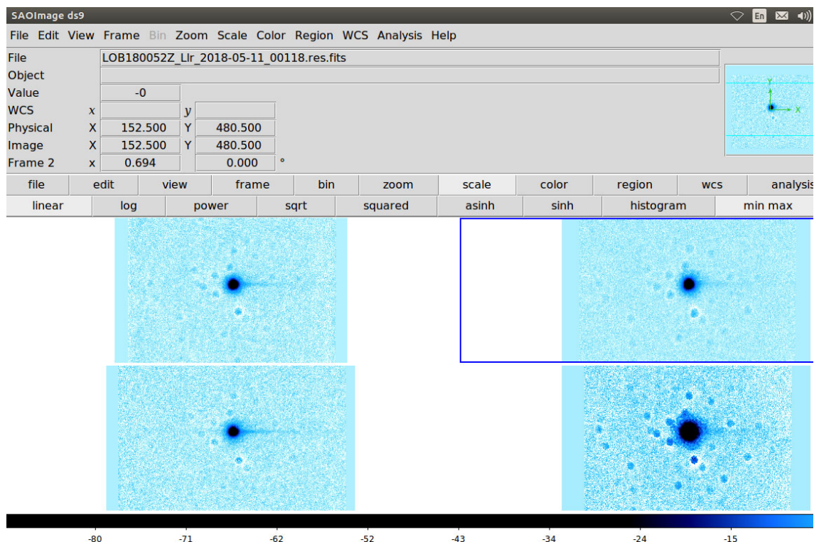
شکل ۴. (رنگی در نسخه الکترونیکی) ۴ نمونه از تصاویر باقی مانده (تصاویر واقعی که از مدل ساخته شده بر مبنای کرنل و تصویر مرجع کم شده است). نقاط تاریک تر مربوط به ستارگان متغیر است.
