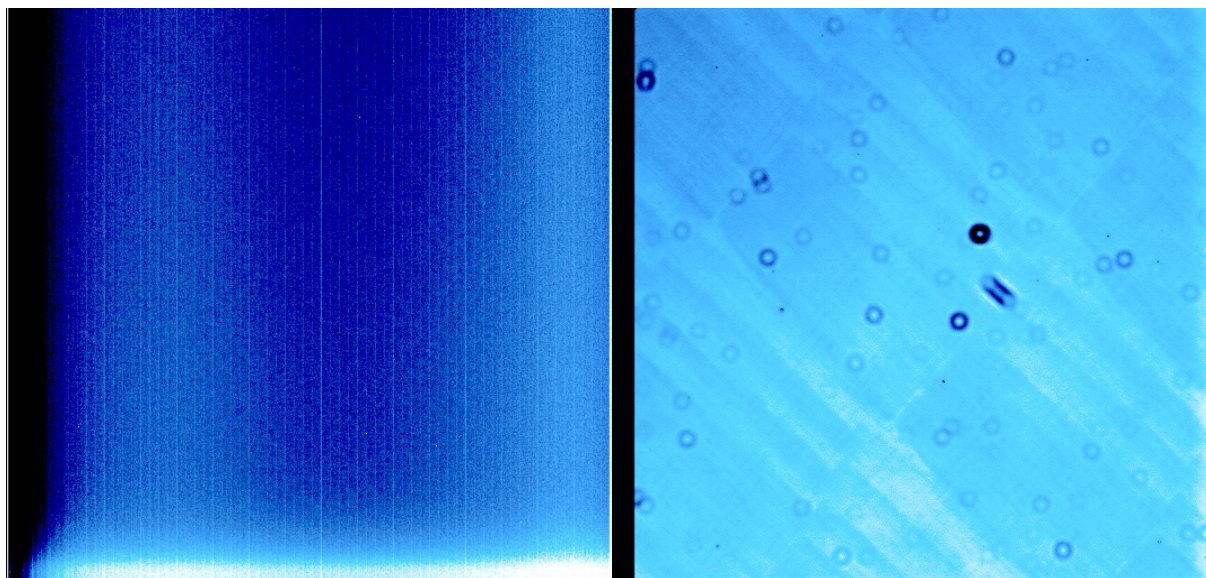
شکل ۲. (رنگی در نسخه الکترونیکی) تصویر سمت راست یک نمونه از یک تصویر هموار و تصویر سمت چپ یک نمونه از یک تصویر سوپیده که به وسیله تلسکوپ دانمارک گرفته شده‌اند، را نشان می‌دهند.
