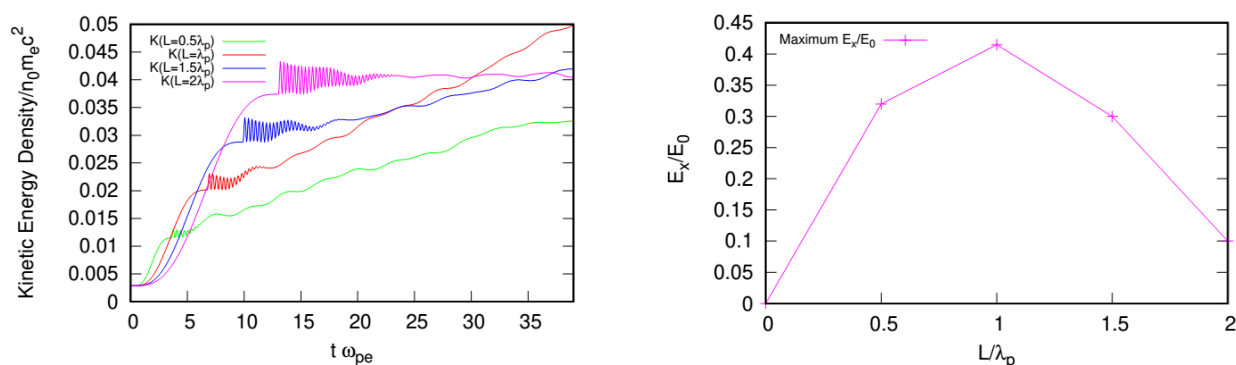
شکل ۵. حداکثر دامنه میدان دنباله‌ایجاد شده پشت پالس لیزر با پوش نیم‌سینوسی بر حسب طول پالس لیزر L . شکل ۶. تحول زمانی چگالی انرژی جنبشی الکترون‌های پلاسما در اثر انتشار پالس‌های لیزر به طول‌های متفاوت L = 0.5\lambda_p ، L = \lambda_p ، L = 1.5\lambda_p و L = 2\lambda_p اما با شدت‌های یکسان در تیغه پلاسما.
