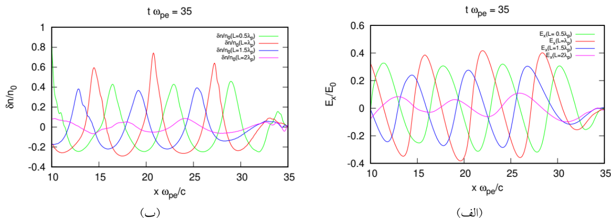
شکل ۴. (الف) میدان الکتریکی ایجاد شده و (ب) تغییرات چگالی در اثر انتشار پالس‌های لیزر به طول‌های متفاوت L = 0.5\lambda_p ، L = \lambda_p ، L = 1.5\lambda_p و L = 2\lambda_p اما با شدت‌های یکسان در تیغه پلاسما.
