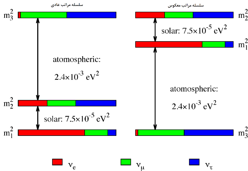
شکل ۲. سلسله مراتب جرم عادی و معکوس نوترینوی دیراک. اختلاف جرم بین نوترینوها توسط آزمایش‌های نوترینوی اتمسفری و خورشیدی به دست آمده است. با توجه به این مقادیر، دو سلسله مراتب محتمل در شکل رسم شده‌اند. در بخش قبل گفتیم که حالت‌های نیروی ضعیف (ویژه حالت‌های طعم) ترکیب خطی از ویژه حالت‌های جرم و برعکس هستند. قسمت‌های رنگی در شکل، میزان مشارکت هر طعم نوترینو در ویژه حالت جرم را نشان می‌دهد [۲۹].
