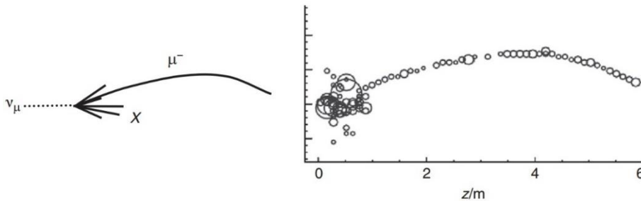
شکل ۳. یک برهمکنش ضعیف جریان باردار (برهمکنشی که ذره واسطه آن بوزون‌های باردار W^\pm هستند). در \nu_\mu + N \rightarrow \mu^- + X آشکارساز آزمایش MINOS. اندازه دایره‌ها نشان دهنده شدت نور تولید شده است. تکانه از طریق میزان انحنایی که میون باردار در میدان مغناطیسی پیدا می‌کند، مشخص می‌شود. همچنین میزان انرژی سیستم هادرونی را با استفاده از مقدار نوری که در رأس برهمکنش تولید شده است، مشخص می‌کنند [۱۵].
