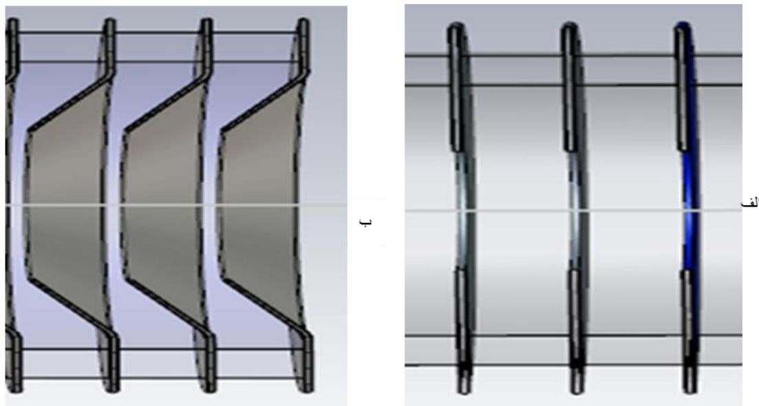
شکل ۴. (الف) الکتروود شتابدهی تخت و (ب) الکتروود شتابدهی لبه دار.
