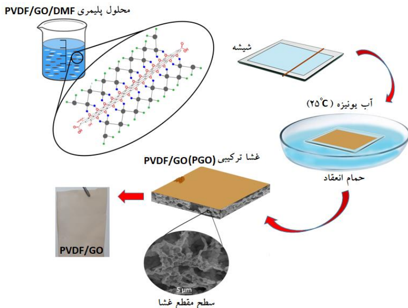
شکل ۱. مراحل ساخت غشاهای PVDF و PGO به روش تبدیل فازی- غوطه‌وری در آب.
