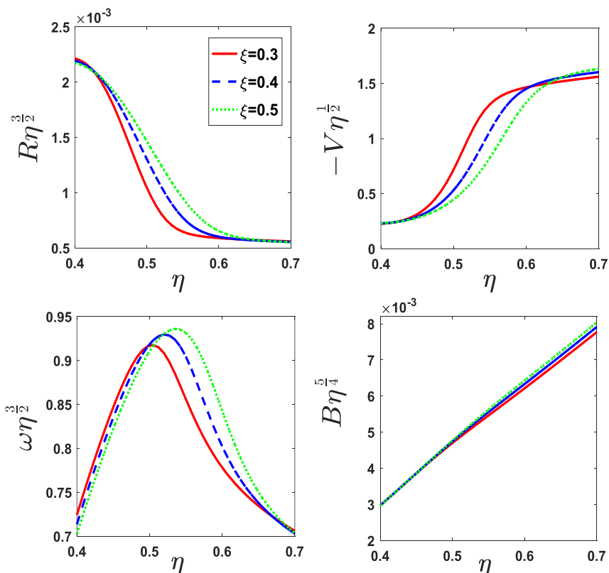
شکل ۳. (رنگی در نسخه الکترونیکی) راه حل‌های خودمشابهی وابسته به زمان m = 0.01 , f = 0.07 , \beta = 0.01 , \alpha = 0.06 و \gamma = 1/33 . خط پر رنگ (رنگ \xi = 0.3 )، خط چین (رنگ \xi = 0.4 ) و خط نقطه چین (رنگ \xi = 0.5 ) اثرات وشکسانی شعاعی را روی کمیات چگالی، سرعت شعاعی، سرعت چرخشی و میدان مغناطیسی نشان می‌دهد.
