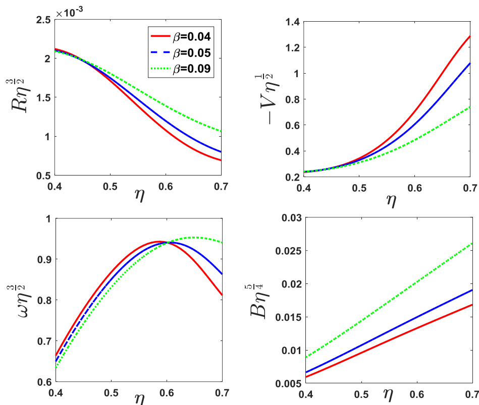
شکل ۱. (رنگی در نسخه الکترونیکی) راه حل‌های خودمشابهی وابسته به زمان \eta برای \alpha = 0.06 ، \xi = 0.09 ، f = 0.07 ، m = 0.01 و \gamma = 1/33 . خط پر رنگ (b = 0.04) ، خط چین (b = 0.05) و خط نقطه چین (b = 0.09) اثرات پارامتر مغناطیسی را روی کمیات چگالی، سرعت شعاعی، سرعت چرخشی و میدان مغناطیسی نشان می‌دهد.
