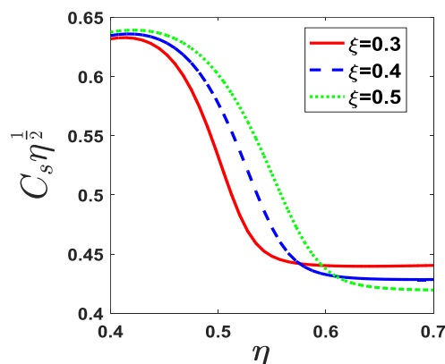
شکل ۴. (رنگی در نسخه الکترونیکی) راه حل‌های خودمشابهی وابسته به زمان m = 0.01 , f = 0.07 , \beta = 0.01 , \alpha = 0.06 و \gamma = 1/33 . خط پر رنگ (رنگ \xi = 0.3 )، خط چین (رنگ \xi = 0.4 ) و خط نقطه چین (رنگ \xi = 0.5 ) اثرات وشکسانی شعاعی را روی دمای قرص نشان می‌دهد.
