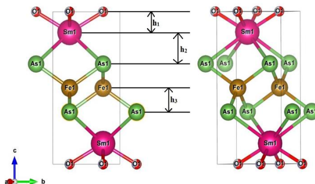
شکل ۴. شبیه‌سازی ساختار بلوری نمونه \text{SmFeAsO}_{0.7}\text{F}_{0.3} .
