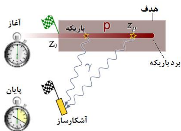
شکل ۱. انتشار پرتو گامای آبی در طی تابش باریکه پروتون.
