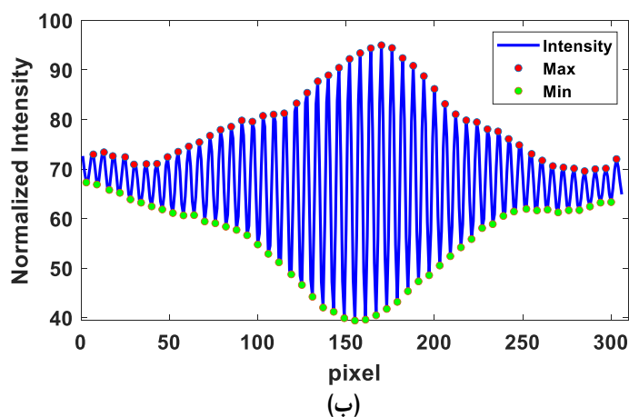
شکل ۴. (الف) تداخل نگاشت ثبت شده توسط طیفسنج، (ب) نمایه یک بعدی شدت و نقاط بیشینه و کمینه جهت محاسبه نمایانی.
