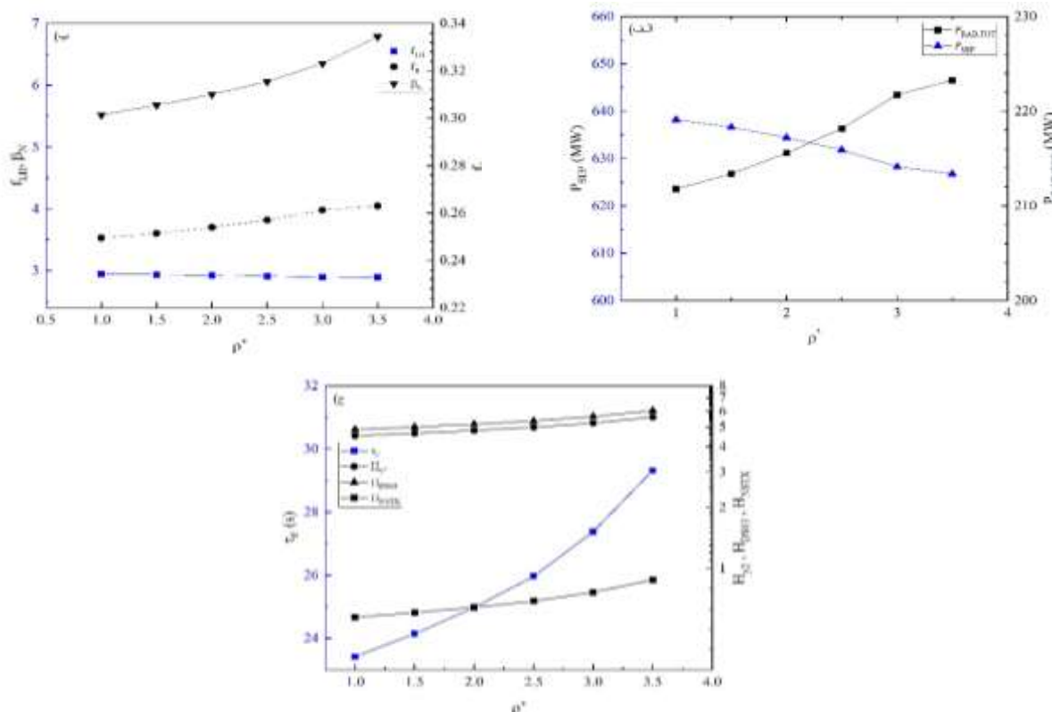
شکل ۲. (الف) توان اتلافی تابش کل P_{rad, TOT} و توان گذرنده از سپرتریکس P_{SEP} بر حسب \rho^* ، (ب) کسر نسبت توان گذرنده از سپرتریکس به توان آستانه f_{LH} ، کسر نسبت توان اتلافی تابش کل به توان گرمایی f_r و بتای بهنجار شده \beta_N نسبت به \rho^* و (ج) زمان محصورسازی انرژی \tau_E بر حسب ثانیه نسبت به \rho^* و ضریب افزایش محصورسازی H بر حسب مقیاس های متفاوت نسبت به \rho^* . همه نمودارها برای توکامک کروی ST در حال سوختن هستند.
