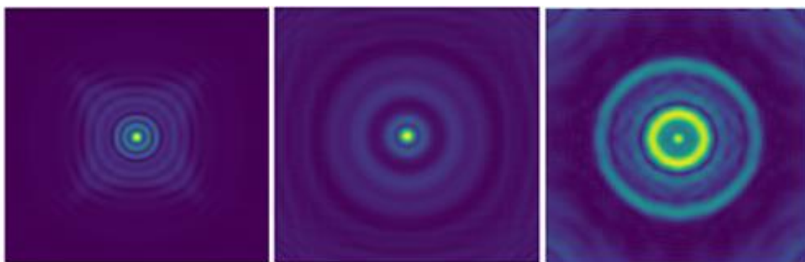
شکل ۹. برش عمودی از الگوی مدهای تشکیل شده در فیبر نوری در دمای 82 درجه سانتی‌گراد. (الف) برش عمودی در انتهای فیبر ( \mu\text{m} ) Z=240 ، (ب) برش عمودی در قسمت مخروطی فیبر ( Z=160 \mu\text{m} ) و (ج) برش عمودی قبل از قسمت مخروطی فیبر ( Z=110 \mu\text{m} ).
