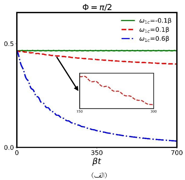
شکل ۴. دینامیک HSS بر حسب تابعی از زمان مقیاس شده \beta t (الف) برای تأثیر اختلاف بسامد قطع باندهای فوتونی متفاوت از بسامد گذار ترازهای بالایی اتم به ازای \phi = \frac{\pi}{2} و (ب) برای مقادیر فاز نسبی اولیه متفاوت \phi ، به ازای \omega_{1c} = -0.1\beta .
