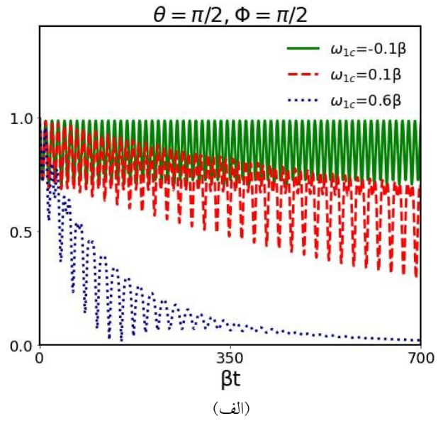
شکل ۳. دینامیک همدوسی کوانتومی بر حسب تابعی از زمان مقیاس شده \beta t (الف) برای اختلاف بسامد گذار تراز بالای اتم از بسامد قطع گاف نواری فوتونی متفاوت به ازای \theta = \frac{\pi}{2} و \phi = \frac{\pi}{2} و (ب) برای مقادیر فاز نسبی اولیه متفاوت \phi ، به ازای \theta = \frac{\pi}{2} و \omega_{1c} = -0.1\beta .
