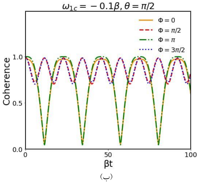
شکل ۳. دینامیک همدوسی کوانتومی بر حسب تابعی از زمان مقیاس شده \beta t (الف) برای اختلاف بسامد گذار تراز بالای اتم از بسامد قطع گاف نواری فوتونی متفاوت به ازای \theta = \frac{\pi}{2} و \phi = \frac{\pi}{2} و (ب) برای مقادیر فاز نسبی اولیه متفاوت \phi ، به ازای \theta = \frac{\pi}{2} و \omega_{1c} = -0.1\beta .
