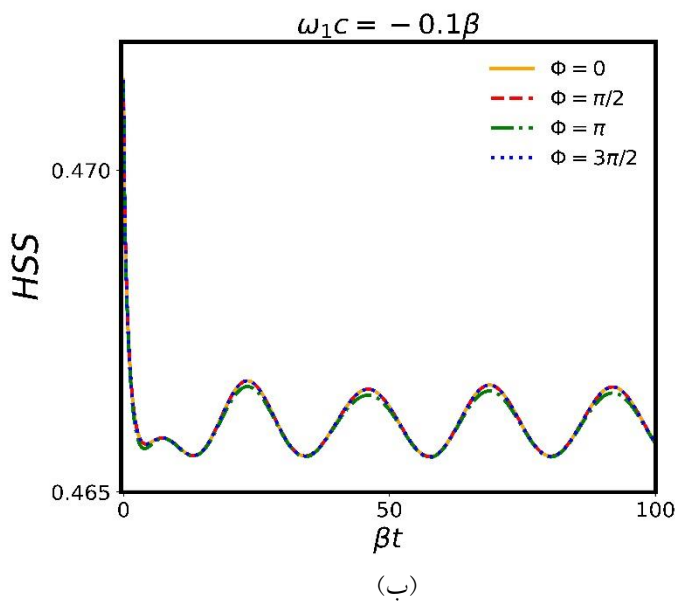
شکل ۴. دینامیک HSS بر حسب تابعی از زمان مقیاس شده \beta t (الف) برای تأثیر اختلاف بسامد قطع باندهای فوتونی متفاوت از بسامد گذار ترازهای بالایی اتم به ازای \phi = \frac{\pi}{2} و (ب) برای مقادیر فاز نسبی اولیه متفاوت \phi ، به ازای \omega_{1c} = -0.1\beta .
