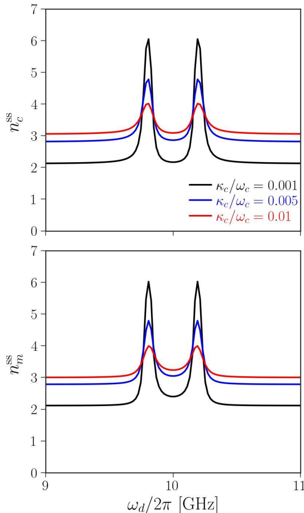
شکل ۳. تعداد فوتون‌ها (سطر بالا) و مگنون‌ها (سطر پایین) در حالت مانا بر حسب بسامد تحریک کاواک \omega_d برای نرخ‌های اتلاف مختلف کاواک که به بسامد کاواک بهنجار شده‌اند.
