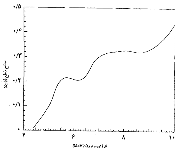
شکل ۱۰. سطح مقطع پراکندگی ناکشسان نوترون با کربن [۴].
