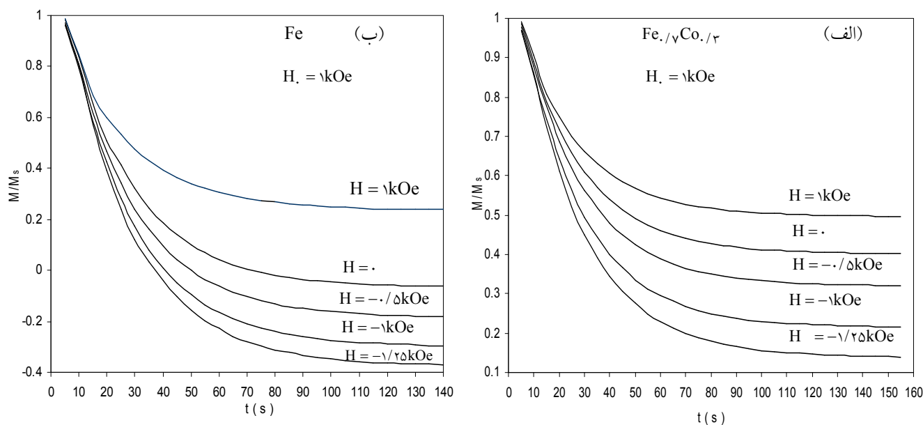
شکل ۸. تغییرات زمانی مغناطش برای دو نمونه (الف) \text{Fe}_{0.7}\text{Co}_{0.3} و (ب) Fe که در حضور میدان H_i = 1/0 \text{ kOe} رشد یافته‌اند.
