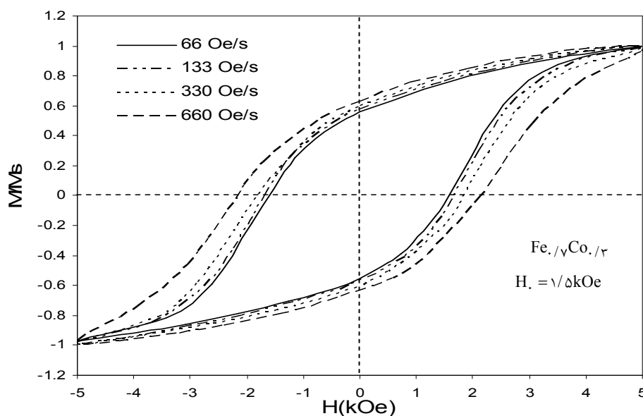
شکل ۷. حلقه های پسماند نمونه \text{Fe}_{0.7}\text{Co}_{0.3} و H_c = 1/5 \text{ kOe} در شرایط تغییر میدان با آهنگهای زمانی متفاوت.
