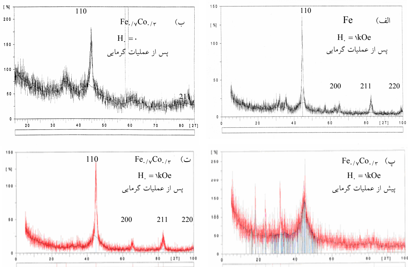
شکل ۲. طیف XRD برای (الف) نمونه Fe پس از رشد در حضور میدان H_c = 1 \text{ kOe} و با عملیات گرمایی، (ب) نمونه \text{Fe}_{0.7}\text{Co}_{0.3} پس از رشد در (ت) نمونه \text{Fe}_{0.7}\text{Co}_{0.3} پس از رشد در حضور میدان H_c = 1 \text{ kOe} و بدون عملیات گرمایی، (پ) نمونه \text{Fe}_{0.7}\text{Co}_{0.3} پس از رشد در حضور میدان H_c = 1 \text{ kOe} و با عملیات گرمایی. برای تمام نمونه‌ها طول موج اشعه ایکس به کار رفته 1.54 \text{ \AA} می‌باشد.
