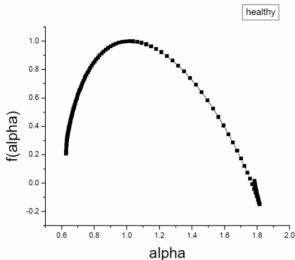
شکل ۳. نمودار طیف تکنیگیاها (singularities) برای سری زمانی سیگنالهای الکتریکی قلب. طیف تکنیگیاها برای یک سیستم نشان‌دهنده میزان پیچیدگی آن است، به این معنی که برای توصیف آن نیاز به تعداد زیادی از پارامترهای مقیاسی داریم. (معادله ۲۲ را ببینید.)
