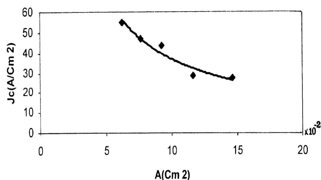
شکل ۴. منحنی J_C - A نمونه YBCO.
