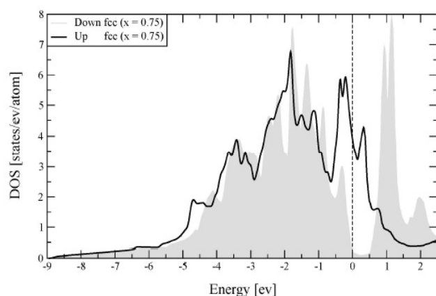
شکل ۳. منحنی چگالی حالت کل آلیاژ \text{Ni}_{0.75}\text{Cr}_{0.25} .
