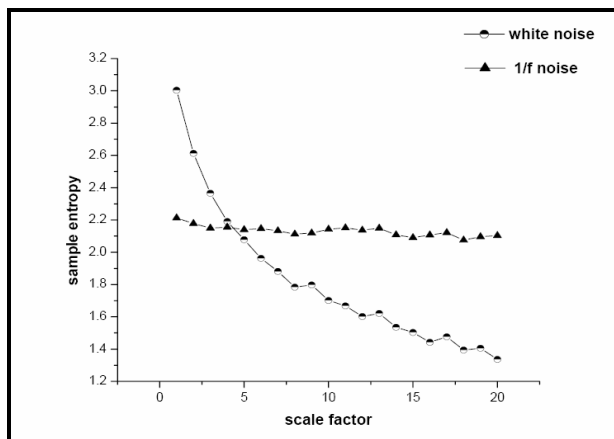
شکل ۳. تمایز نوفه سفید و نوفه ۱/f توسط روش آنتروپی چند مقیاسی.
